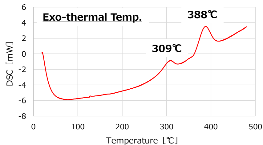
[ DSC-DTA ]
