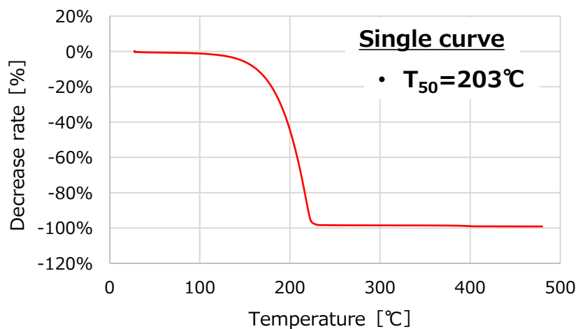
[ TG-DTA ]
